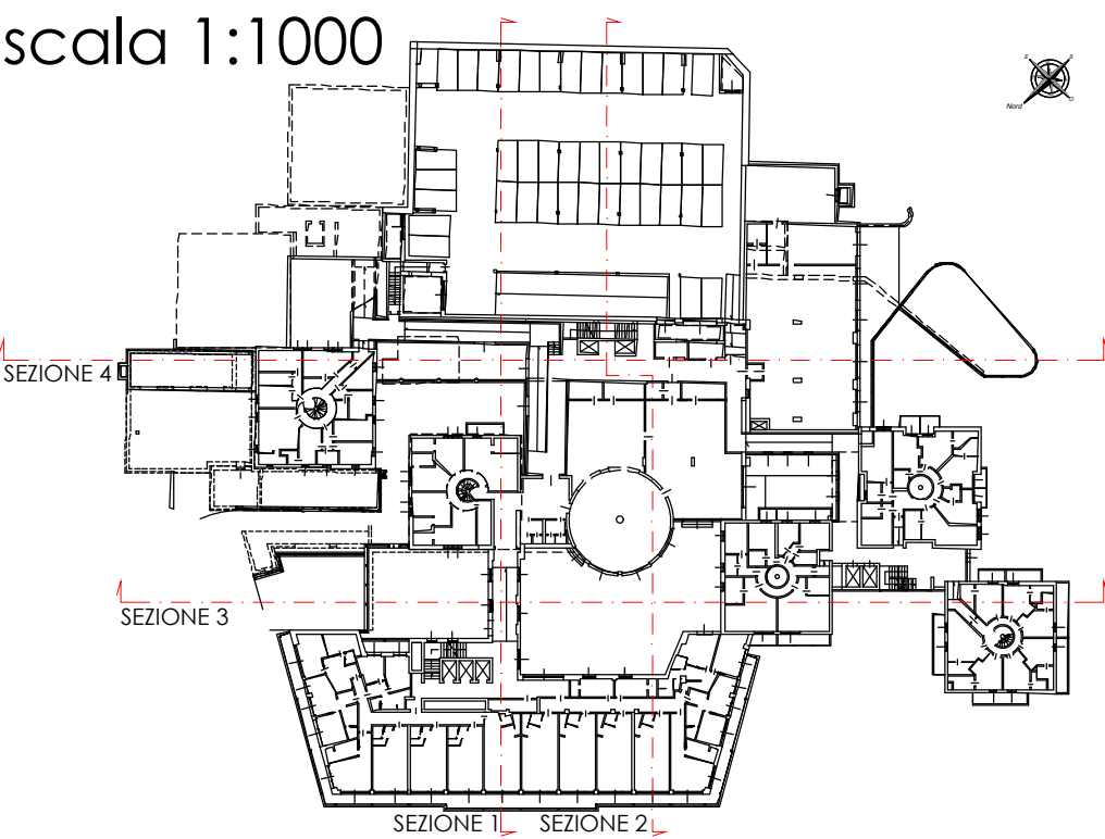
SCHEMA SEZIONI
