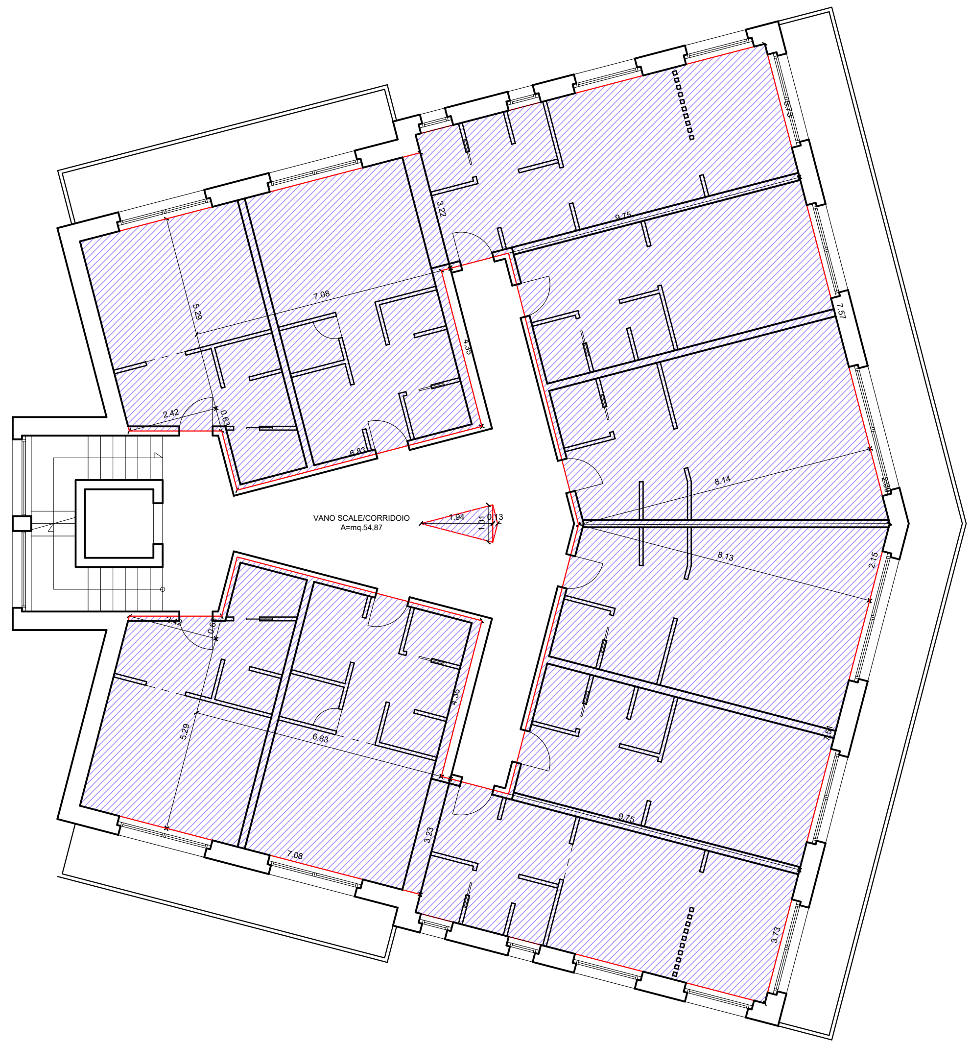
PIANTA PIANO TERZO PROGETTO
