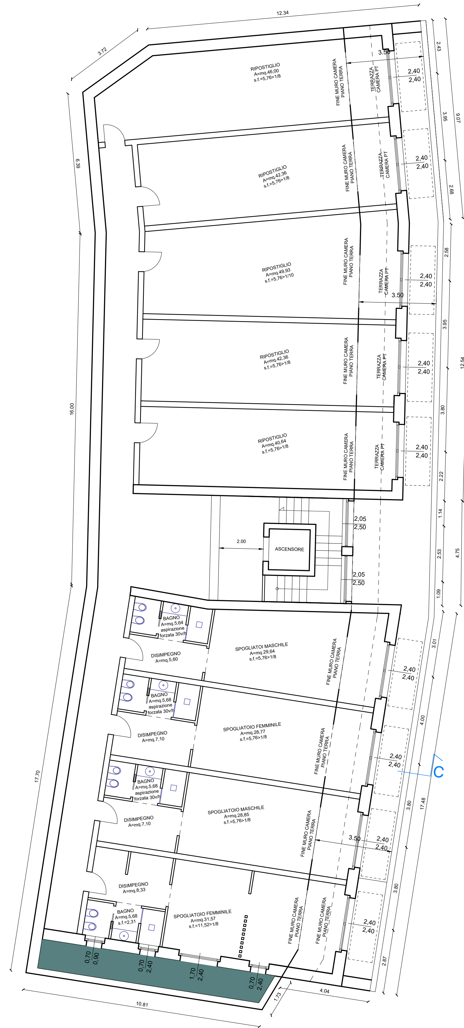
PIANTA PIANO SEMINTERRATO 2 PROGETTO
