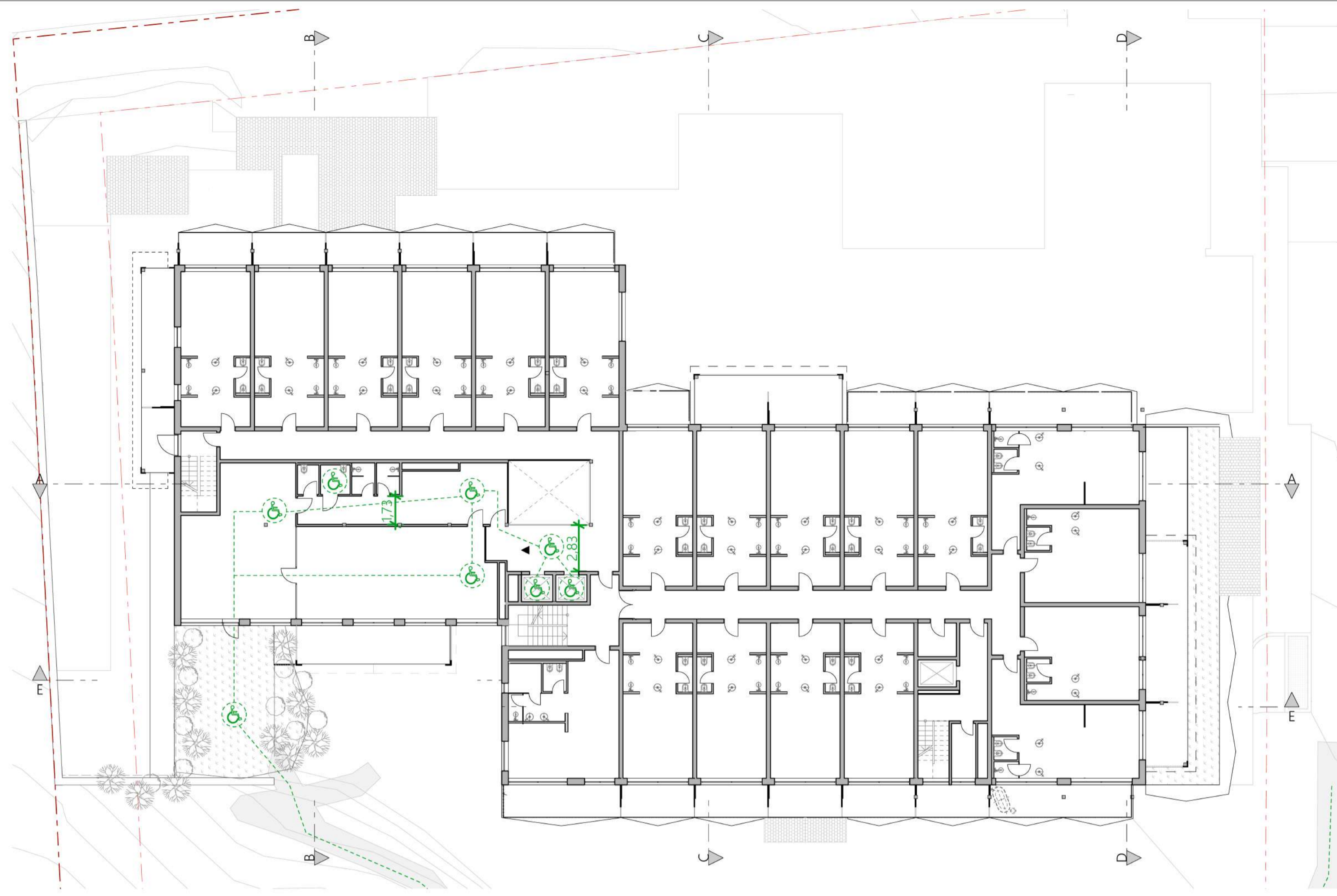
2. Piano - Barriere architettoniche
