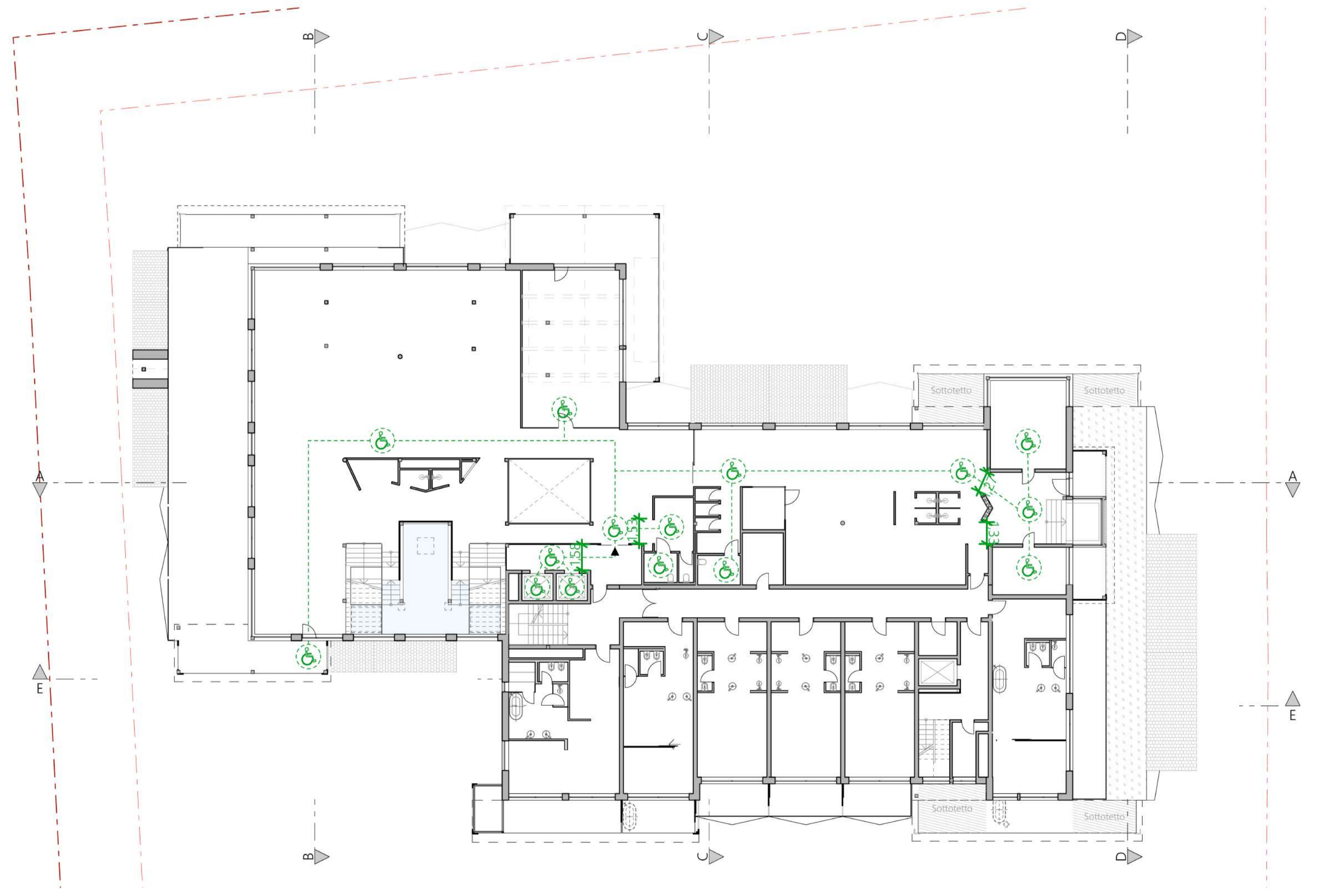
4. Piano - Barriere architettoniche
