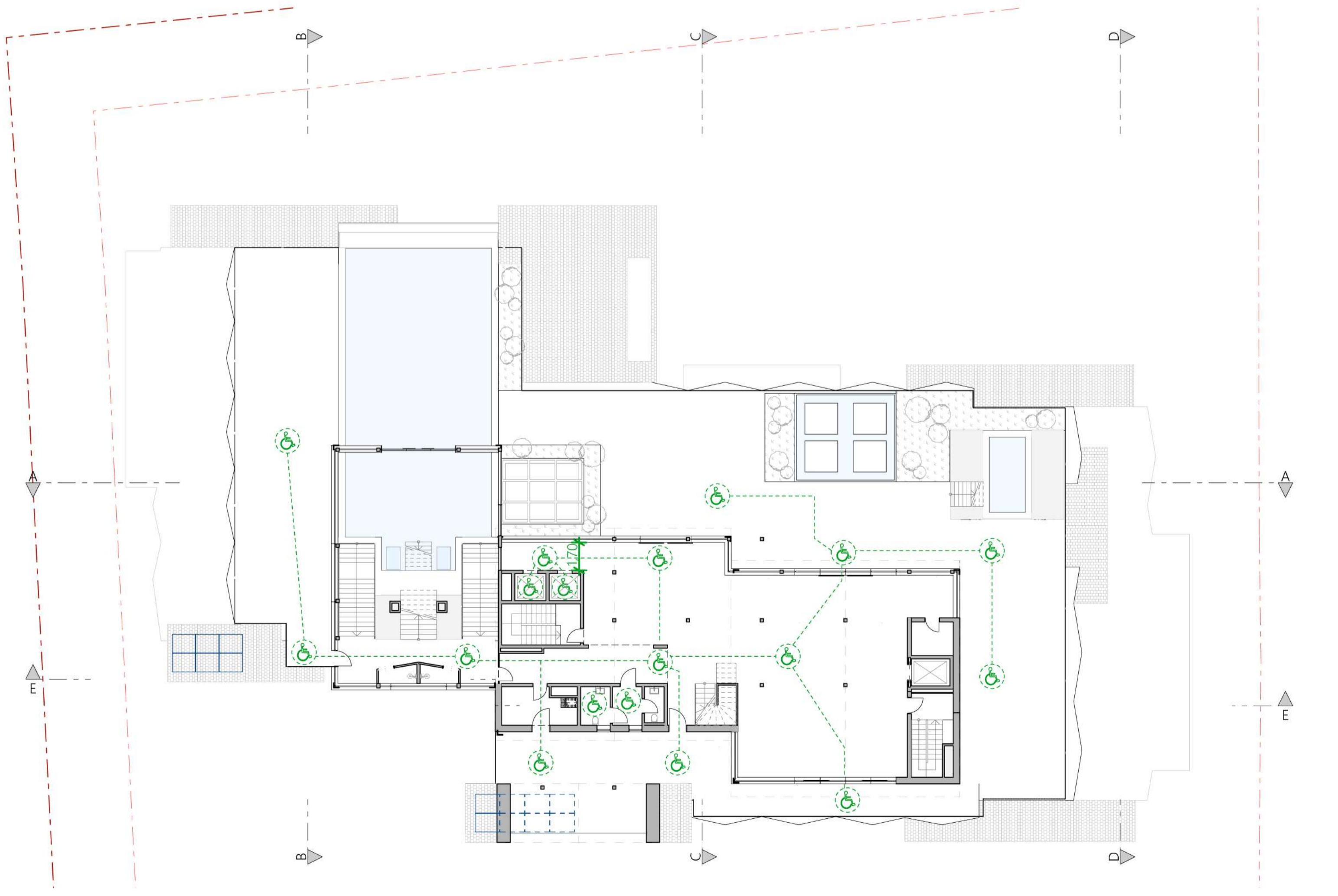
5. Piano - Barriere architettoniche
