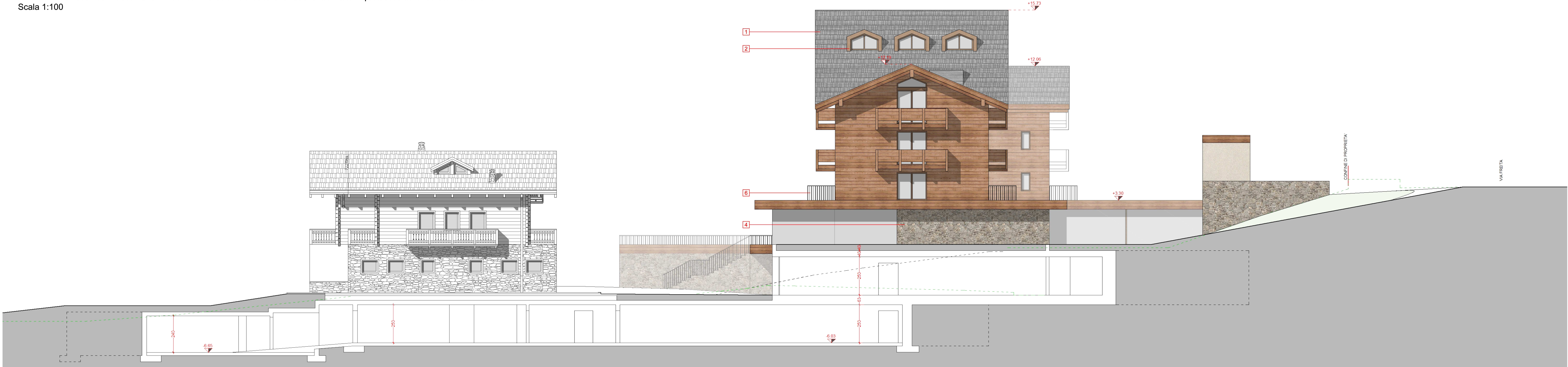
PROSPETTO NORD/SEZIONE C-C' - VARIANTE Scala 1:100
